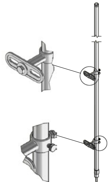
0227-480 Tube à eau pour le nourrisseur COMBI
